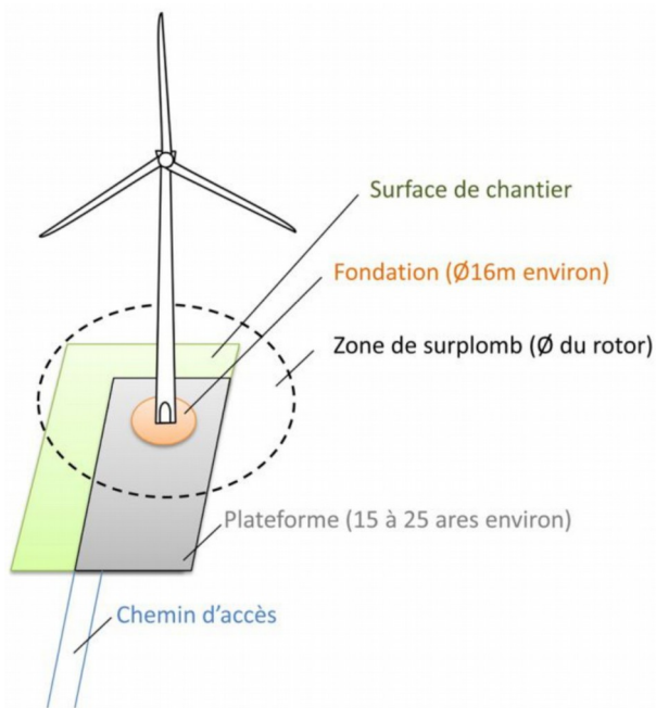
Illustration 2: Illustration des emprises au sol d'une éolienne
